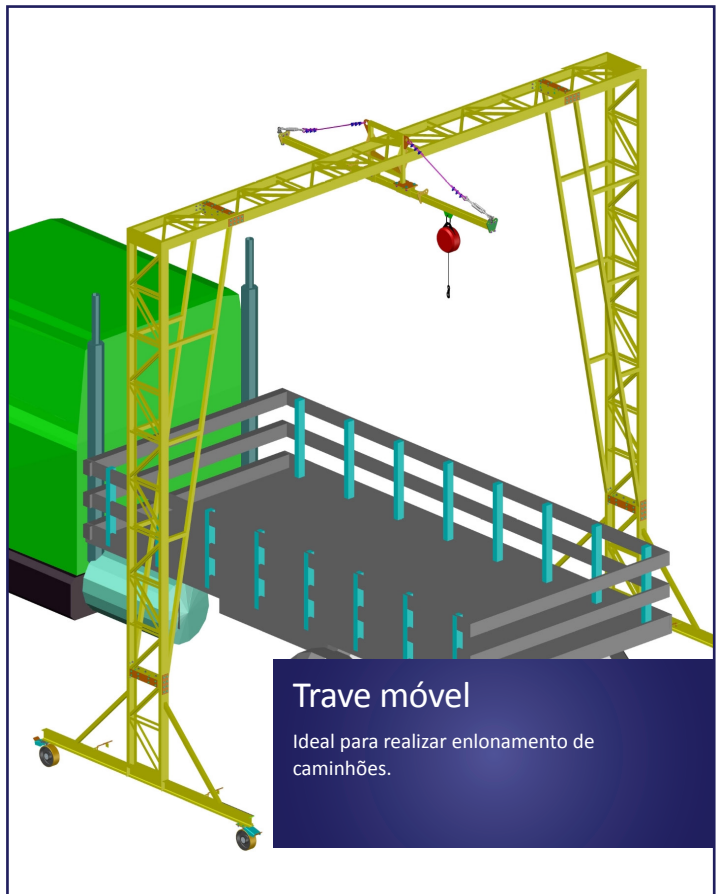
Linha de vida abraçada em estrutura existente Pode ser ajustada para se adaptar a desníveis ou desviar de interferências.
