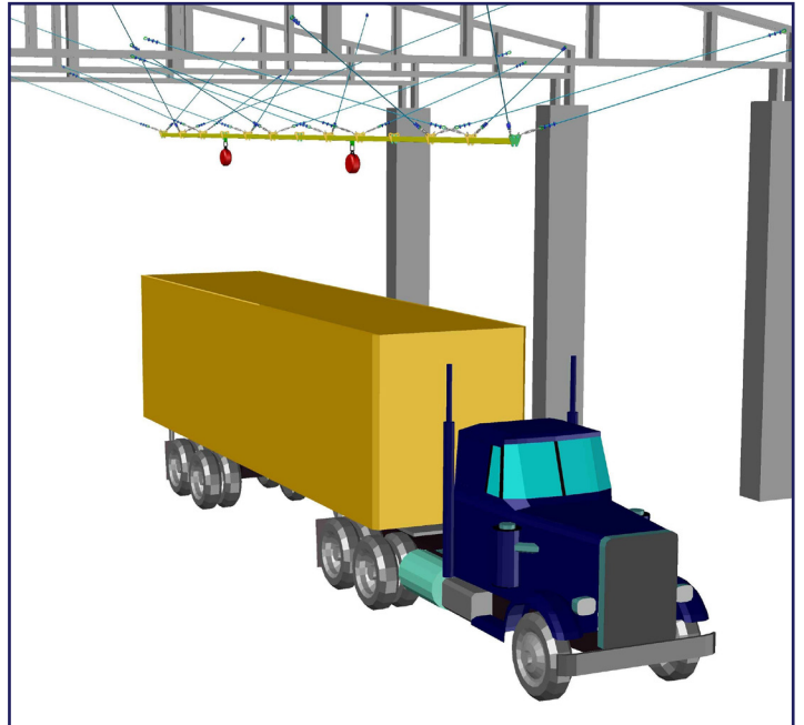
Linha de vida atrantada em telhado existente Composta pelo trilho e cabo de aço, criando um sistema seguro e estável.
